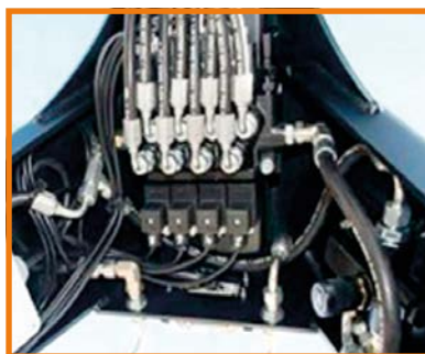
Distributore proporzionale (2)
